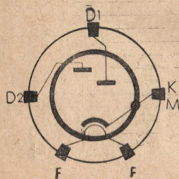
Sockelschaltung
